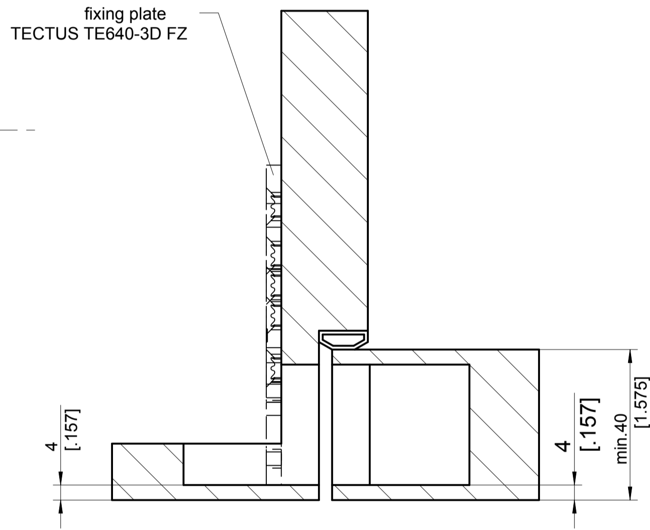
template door panel
