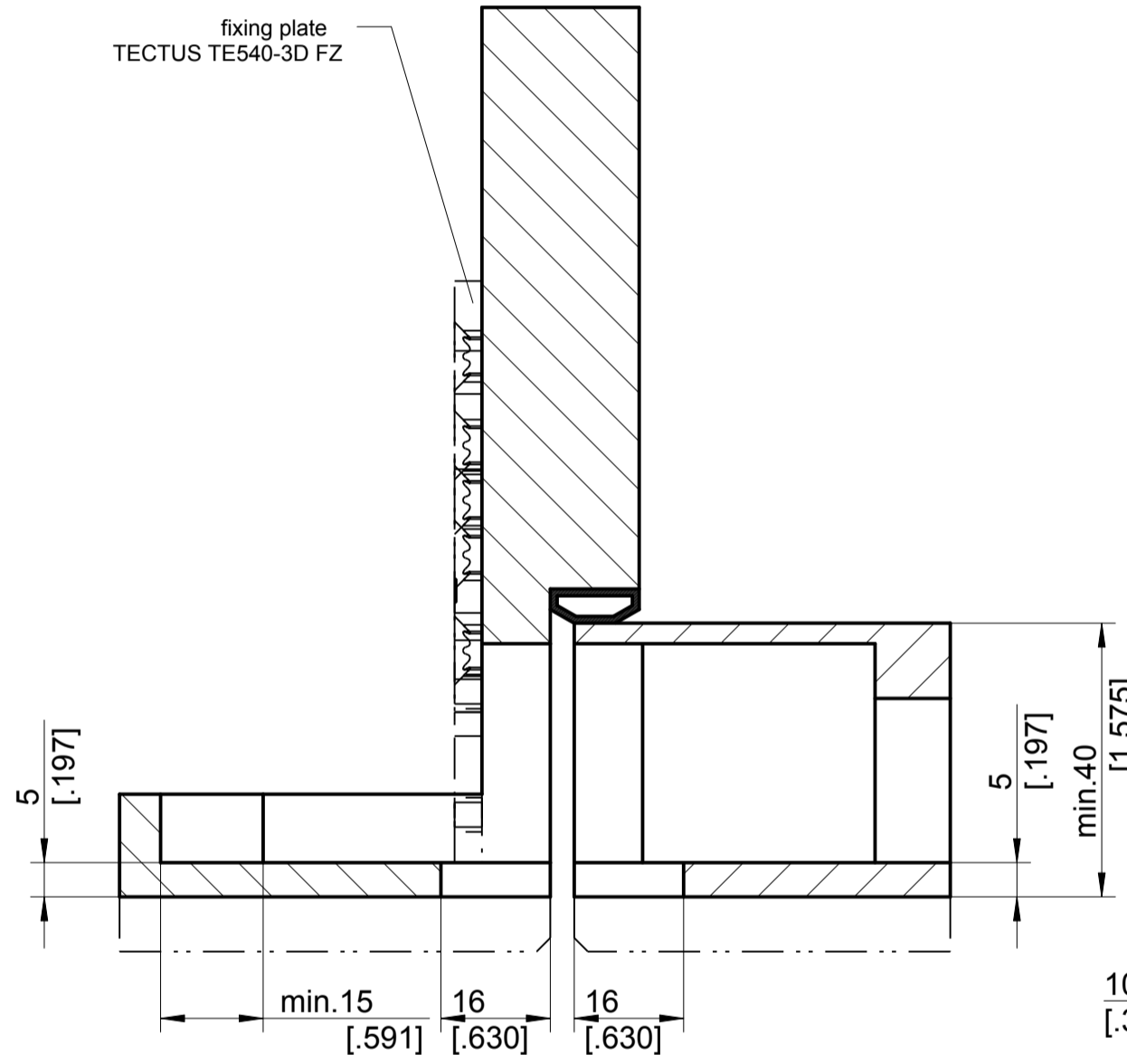
template door panel
